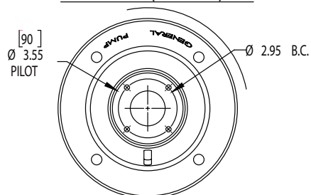
ZF184N (500004)
